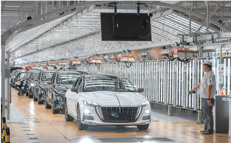
工人在位于吉林长春的一汽红旗繁荣工厂总装车间检查车辆(2023年7月6日摄)。 新华社发
