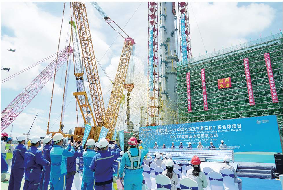
EO/EG洗涤塔吊装成功,现场人员见证历史时刻。
