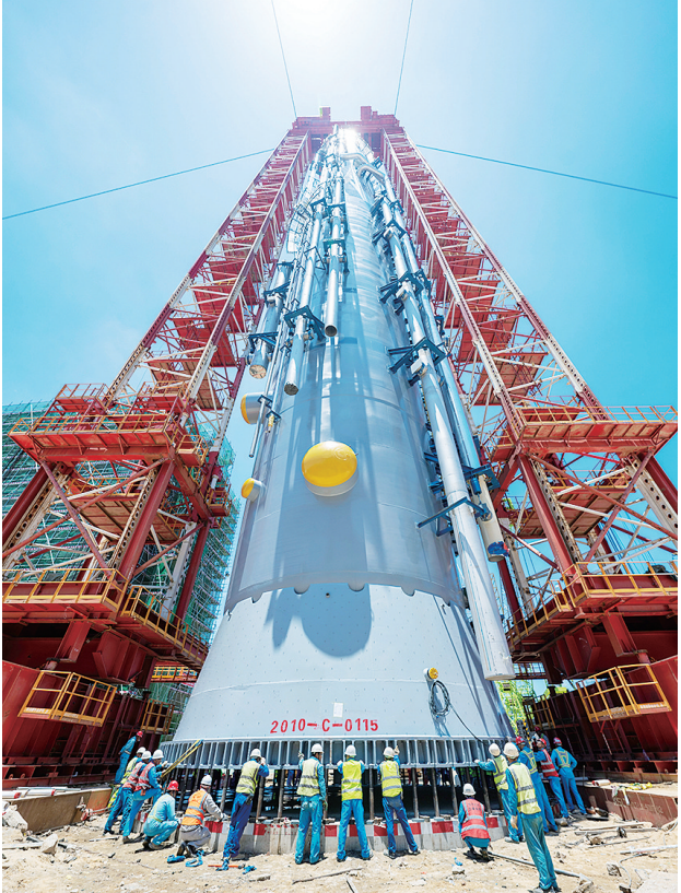
EO/EG洗涤塔缓缓平移至混凝土基座
